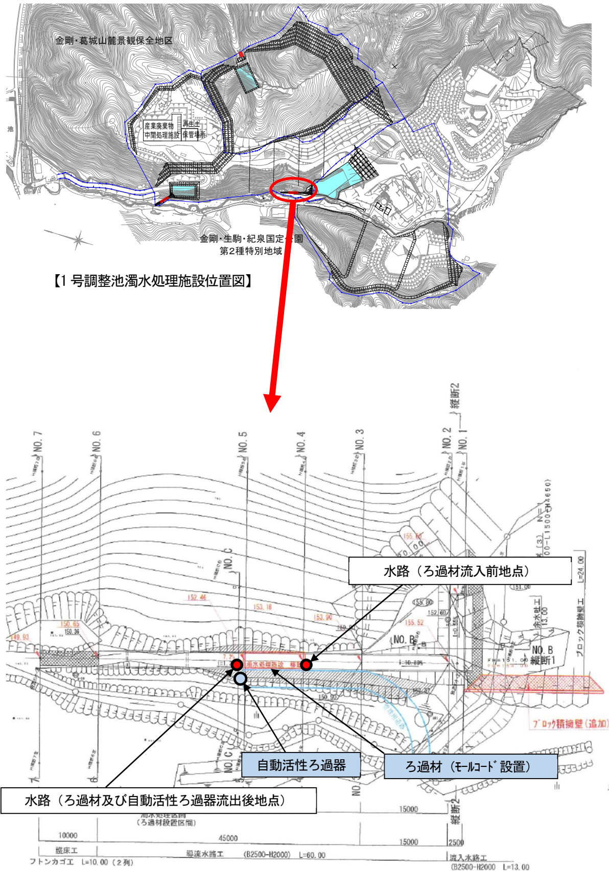
図 1.2 濁水処理施設（ろ過材等）の位置図
